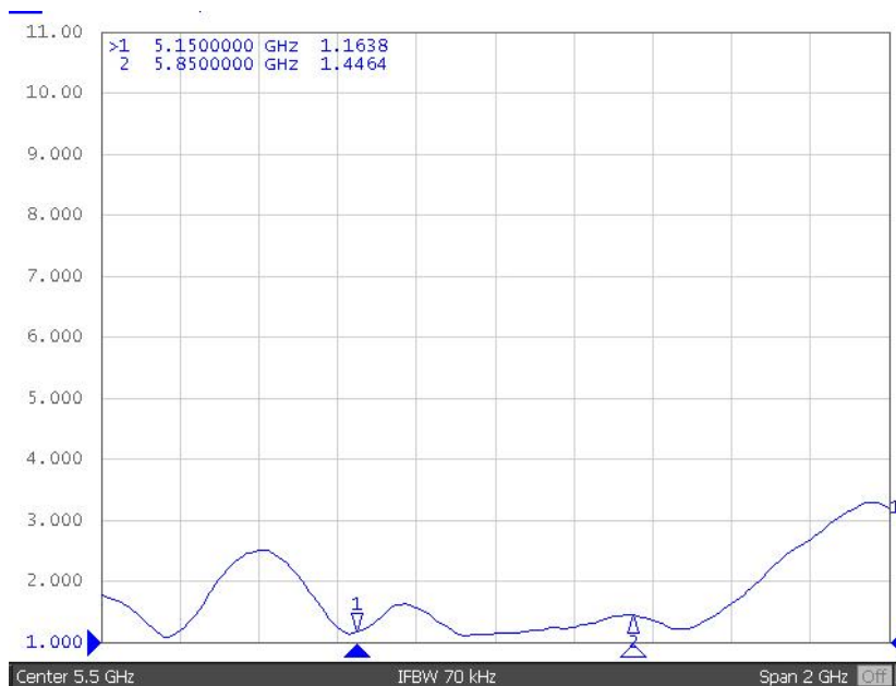
电压驻波比 (VSWR)
