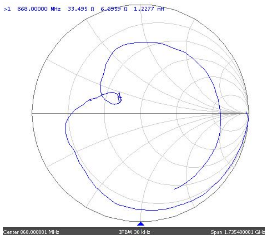
史密斯圆图 (Smith chart)
