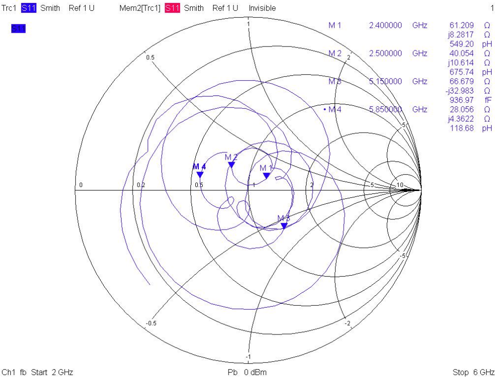
史密斯圆图 (Smith chart)
