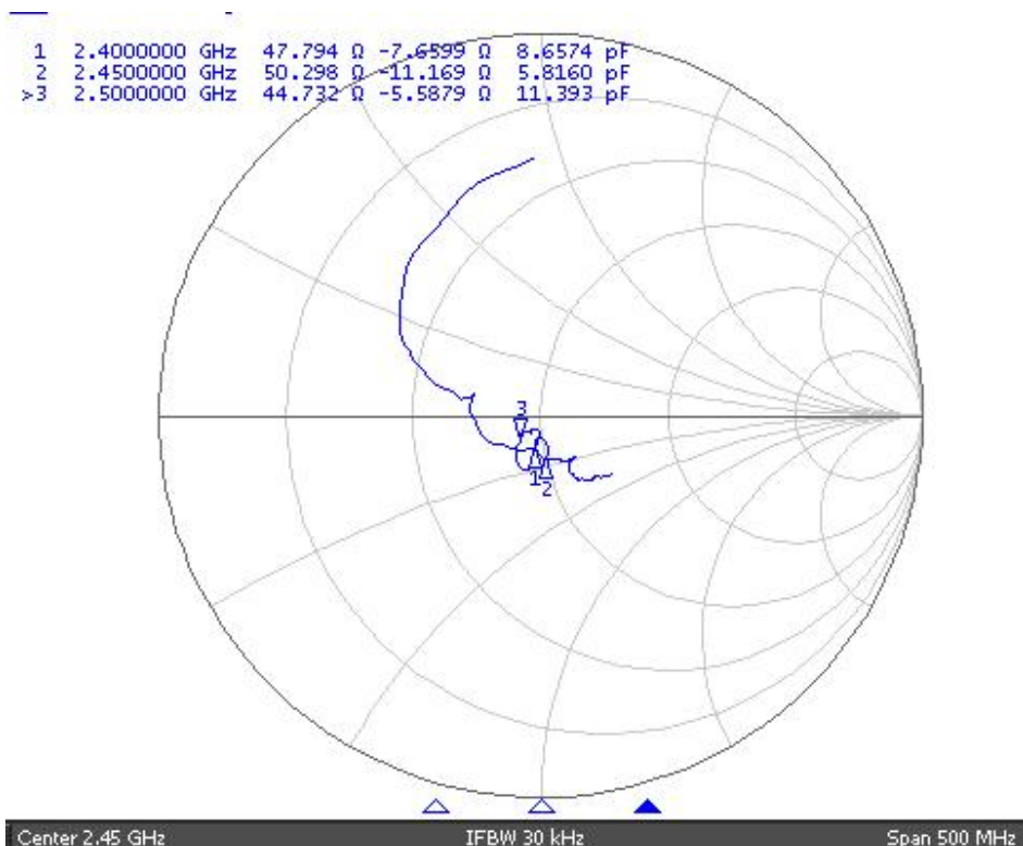
史密斯圆图 (Smith chart)
