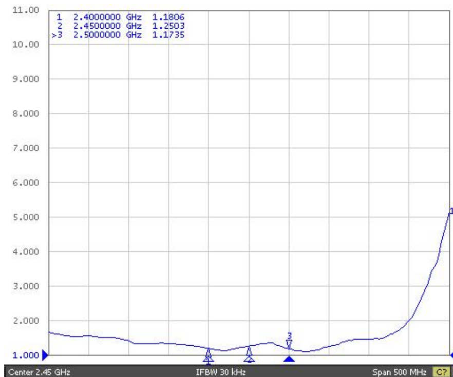
电压驻波比 (VSWR)
