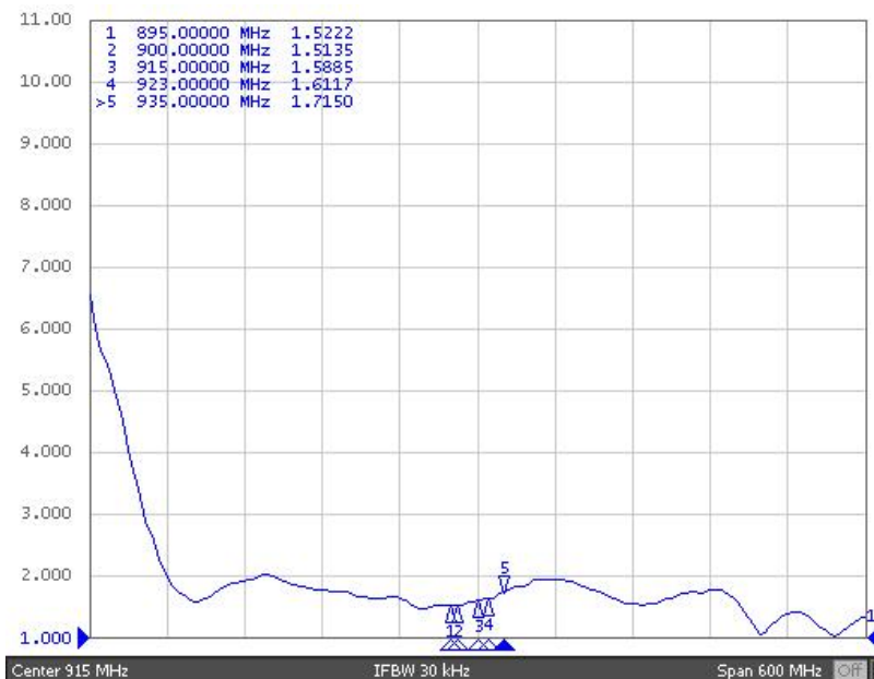
电压驻波比 (VSWR)
